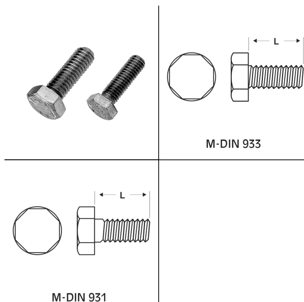
M-DIN 931
