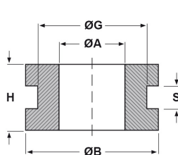
forma piana
