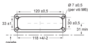
DIMENSIONI FORI PARETE
